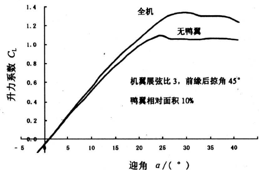
图2 鸭翼对低速最大升力特性的影响 (风洞试验, Ma = 0.2 )
