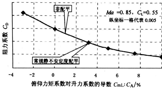
图1 高亚声速稳定盘旋阻力系数随纵向静不稳定性变化趋势
